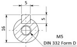
KESİT A-A
